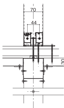
C-C断面詳細図
