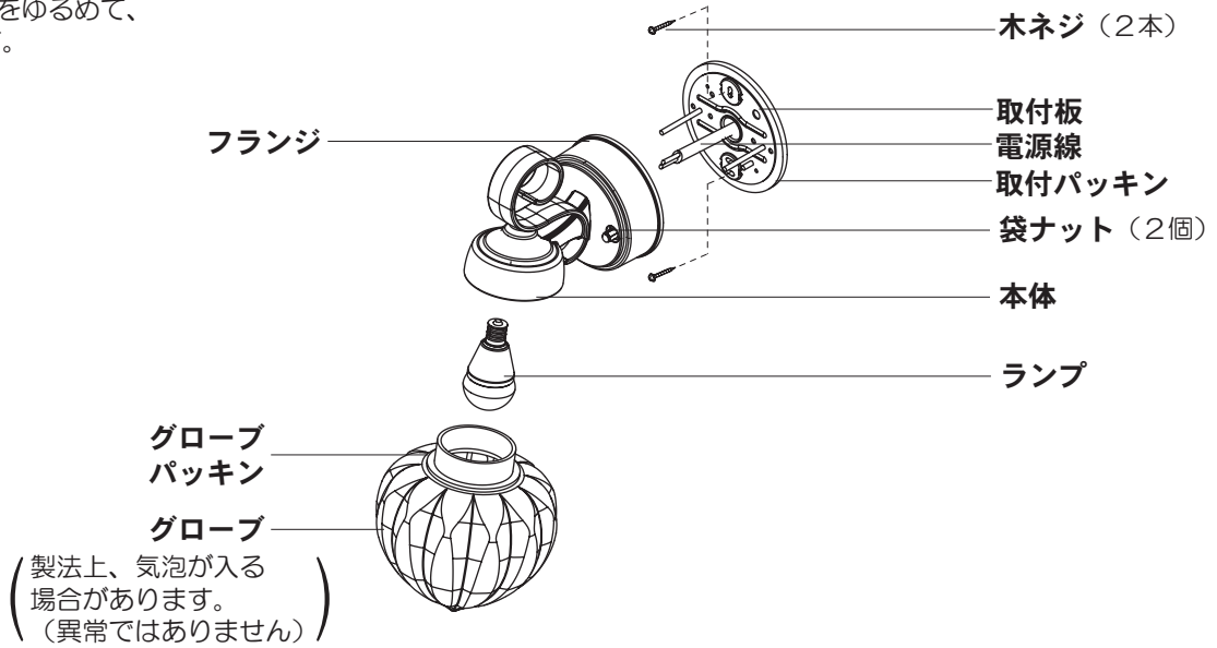
木ネジ (2本)
