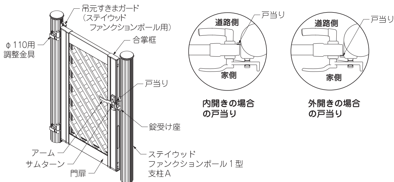
ステイウッドファンクションポール1型（支柱A+ステイウッドB錠仕様）
