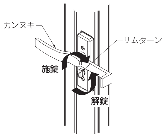
図3-4 サムターンが左側にある場合
