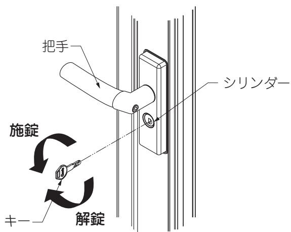
図3-1 シリンダーが左側にある場合
