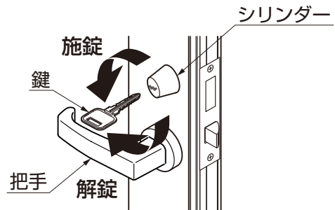
図3-2 シリンダーが左側にある場合
