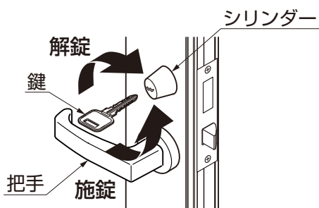
図3-7 シリンダーが左側にある場合
