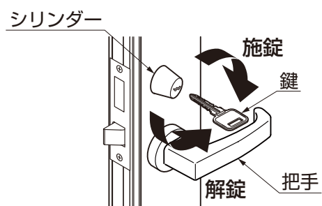
図3-8 シリンダーが右側にある場合
