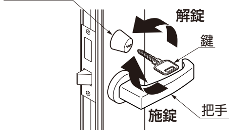
図3-1 シリンダーが右側にある場合
