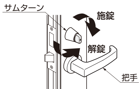
図3-4 サムターンが右側にある場合
