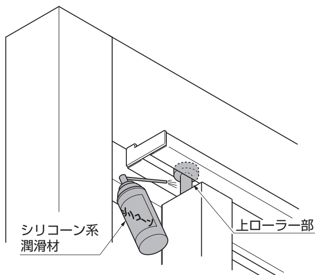
見上げ図
