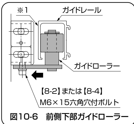
【8-2】または【8-4】 M6×15六角穴付ボルト
