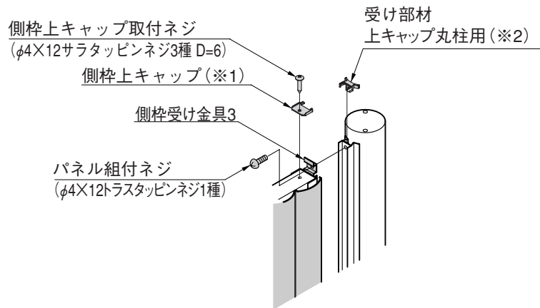
図3-2 丸柱の場合
