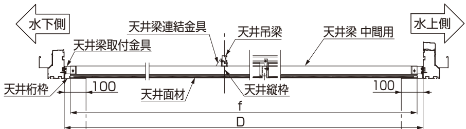
図3-2 B-B断面図
