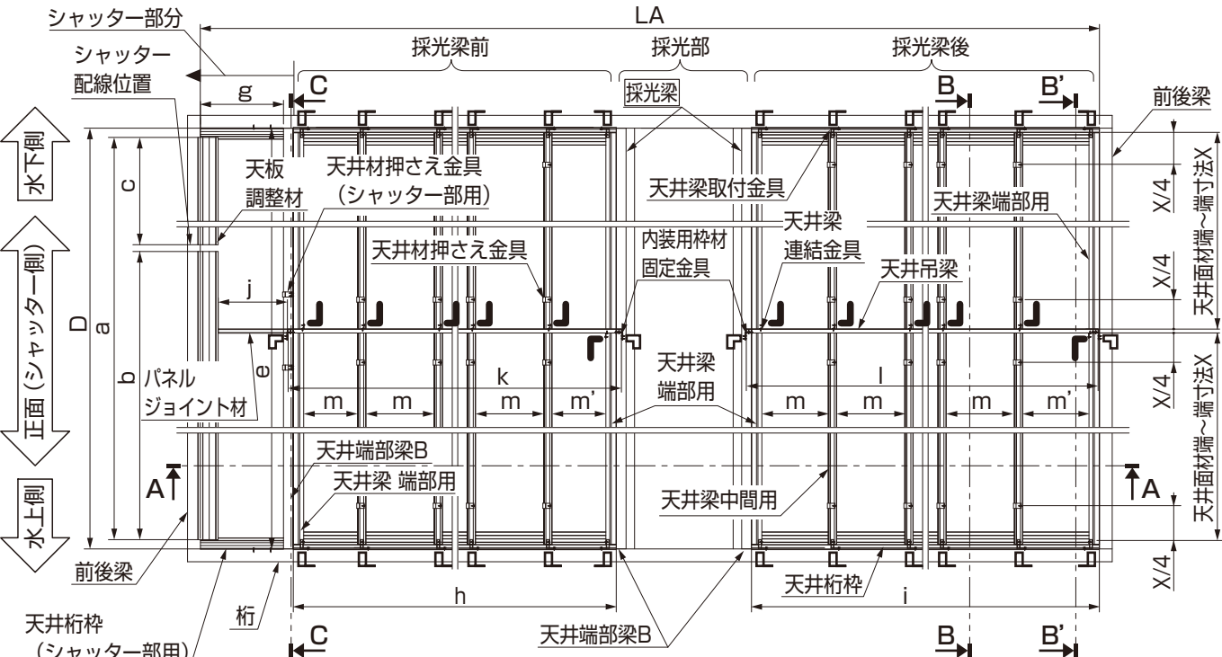
図3-1 上面図
