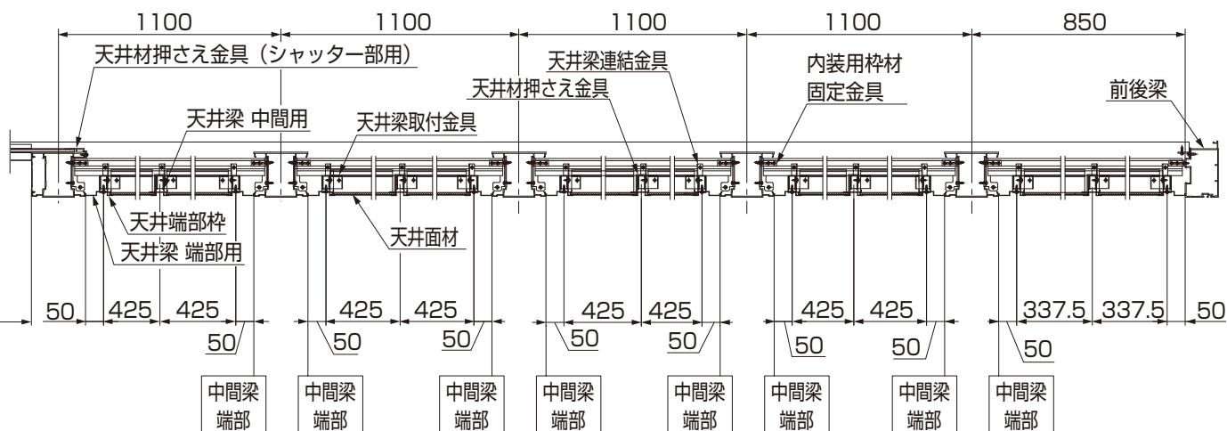
図3-15 A-A断面図
