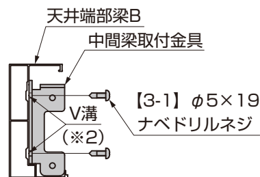
図5-10 中間梁取付金具取付け位置（スタイルコートの場合）
