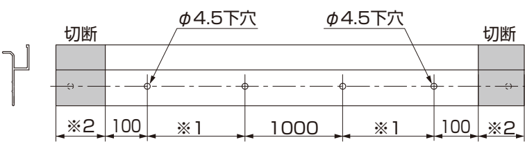
図6-1 天井端部枠加工寸法
