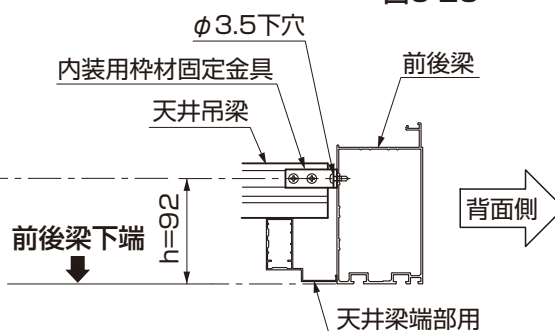
図6-21 スタイルコートの場合の天井吊梁の取付け位置
