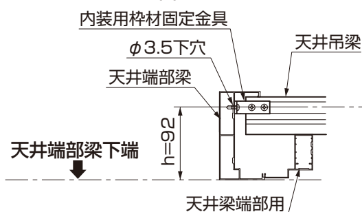
図6-21 スタイルコートの場合の天井吊梁の取付け位置
