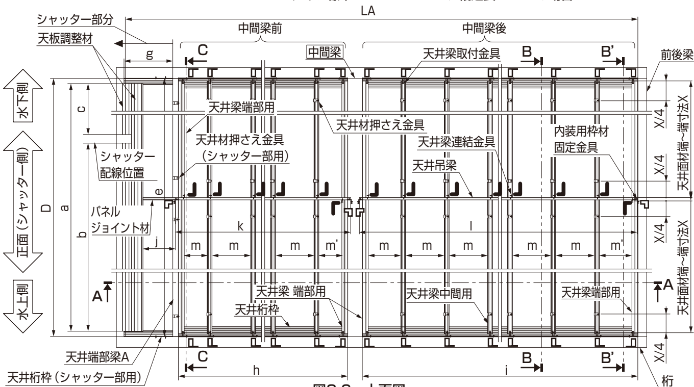
图3-6 上面图
