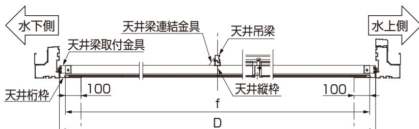
图3-7 B-B断面图
