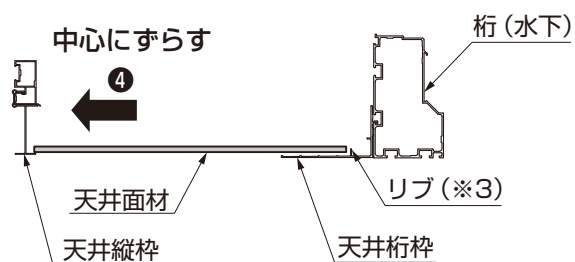
図6-38 天井面材のはめ込み方法 (間口方向)
