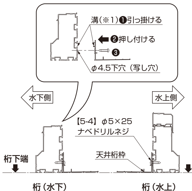
図6-9 スタイルコートの場合
