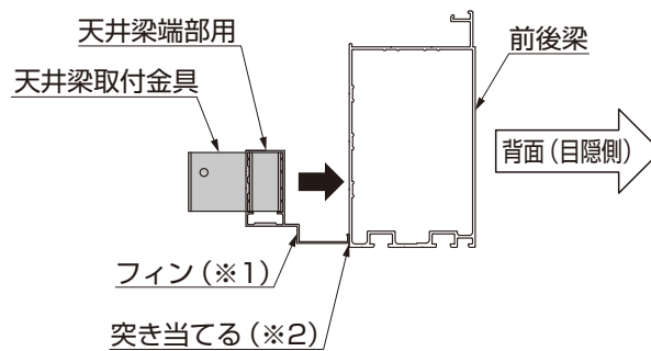
図6-14 天井梁端部用の向き（前後梁側）
