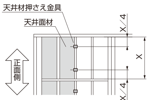
図6-41 天井材押さえ金具の取付け位置
