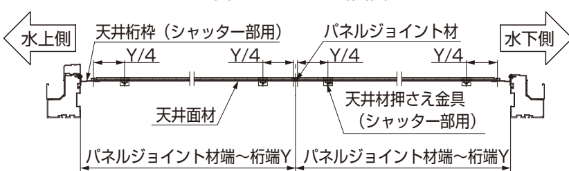
図3-9 C-C断面図(シャッター部分)
