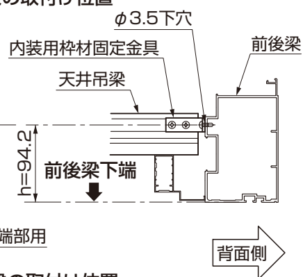
図6-22 スタイルコートLの場合の天井吊梁の取付け位置
