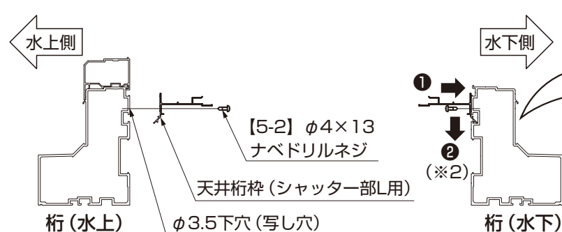
図5-4 スタイルコートLの場合
