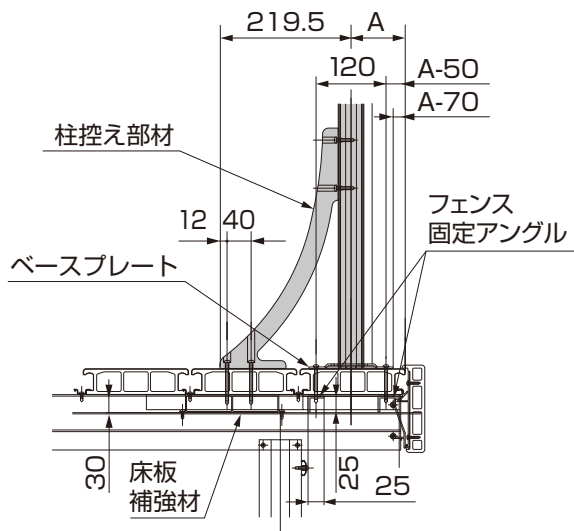
図3-14 A-A矢視図
