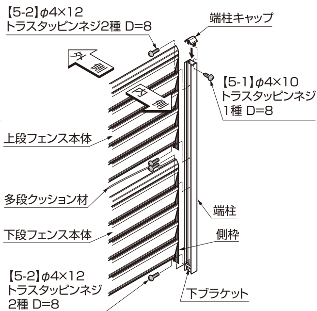
図4-2 端柱の場合
