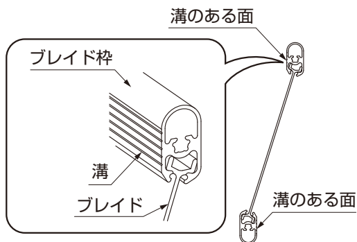
図6-5 ブレイドの挿入
