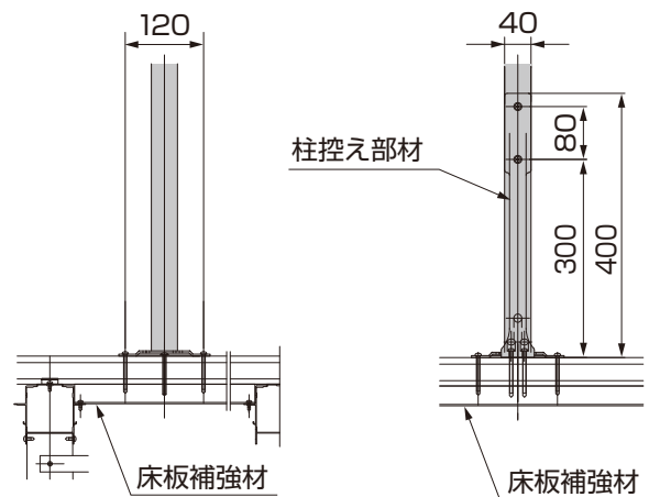
B-B矢視図 図3-20
