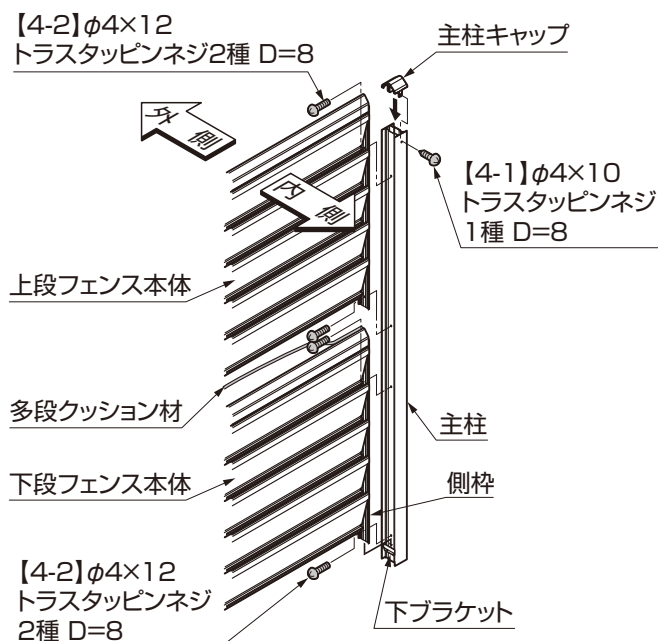
図4-1 主柱の場合
