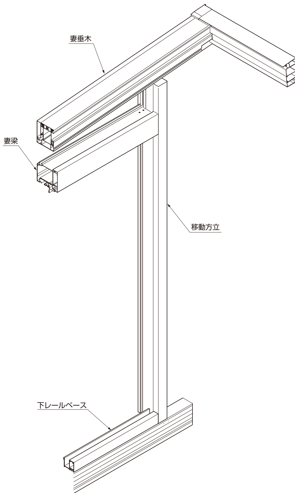
図1-1 妻垂木納まり
