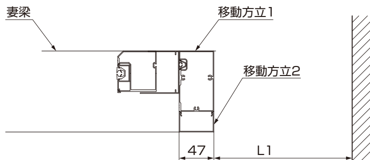
図2-2 移動方立を使用する場合
