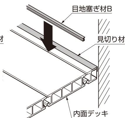
図1-23 入隅タイプ
