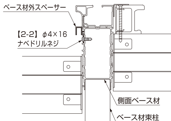
図2-10 側面
