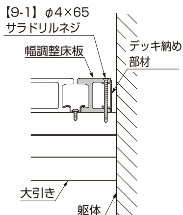
図1-20 入隅タイプ
