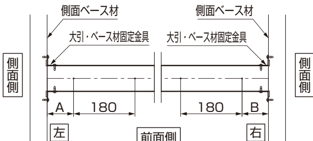
図1-3 大引き平面図(基本仕様)
