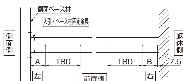
図1-4 大引き平面図(入隅仕様)
