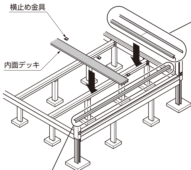
図1-8 基本タイプ
