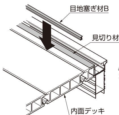
図1-22 基本タイプ
