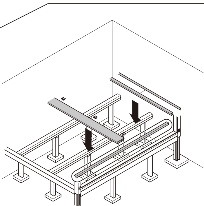
図1-9 入隅タイプ
