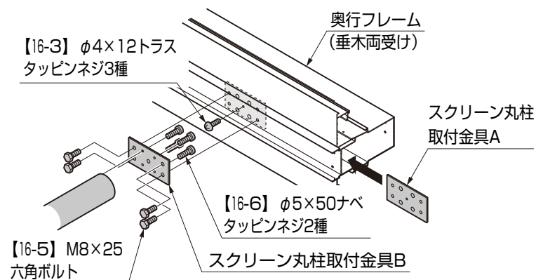
図1-8 両端部の取付け
