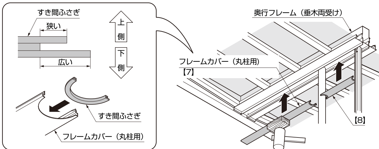
図12-2 フレームカバー (丸柱用) の取付け
