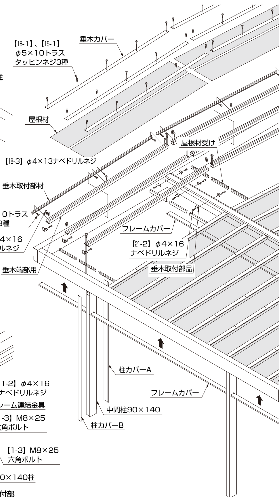
図1-1 端部柱仕様の場合
