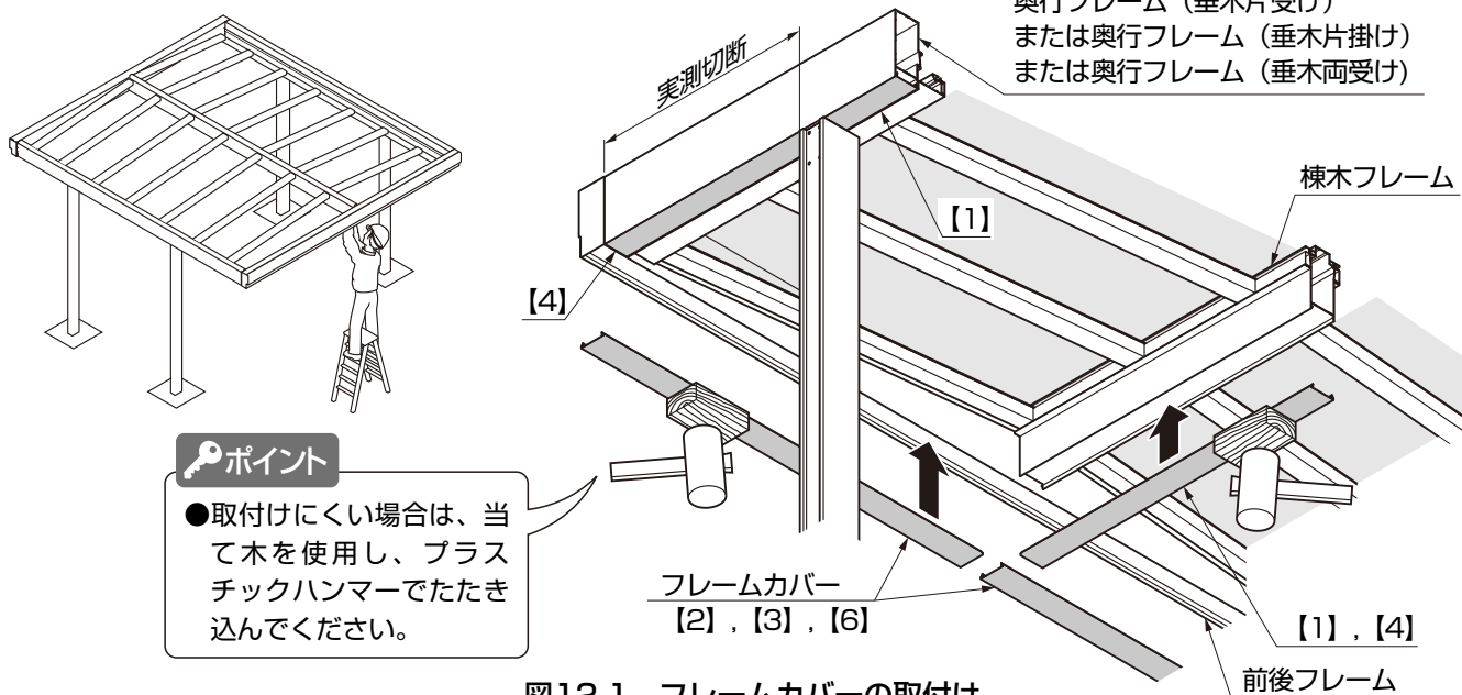
図12-1 フレームカバーの取付け
