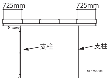
奥行：36 の場合
