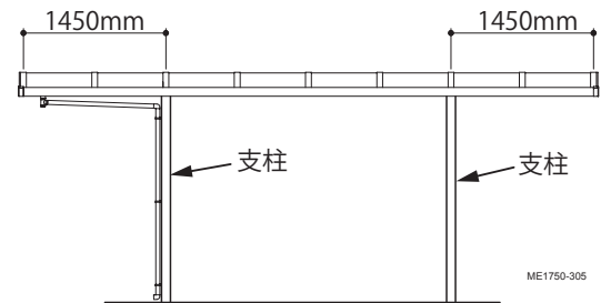
奥行：58 の場合
