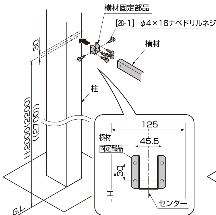
図3-3 角柱の場合
