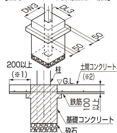
図1-3 8本柱
