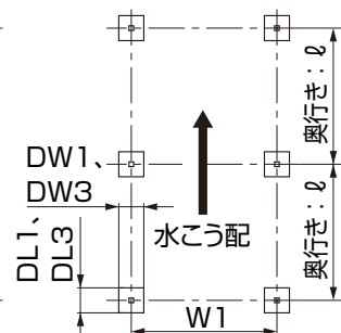
図1-2 6本柱
