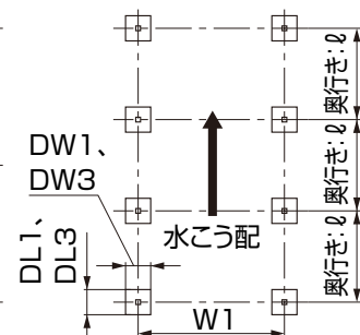
図1-3 8本柱
