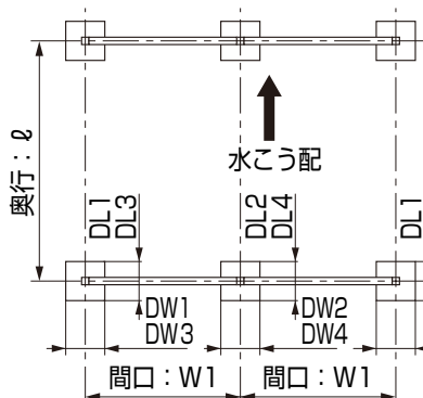
図1-7 横連棟6本柱 幅55+55、幅60+60サイズ
