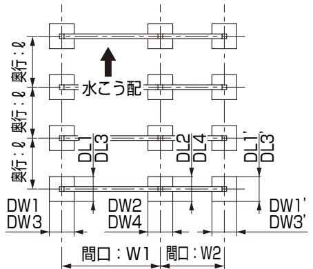
図1-6 横連棟12本柱 幅30+55、幅30+60サイズ
