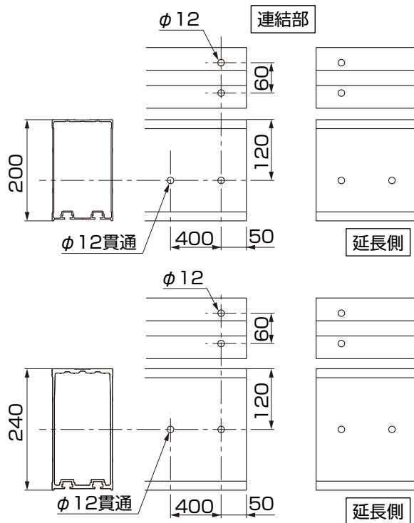
図2-10 幅18延長仕様
