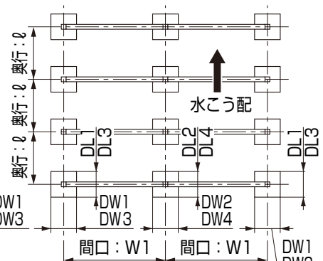
図1-9 横連棟12本柱 幅55+55、幅60+60サイズ
