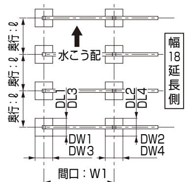
図1-12 幅18延長8本柱 幅55+18、幅60+18サイズ
