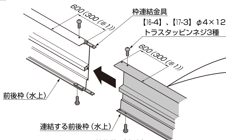
図5-4 前後枠 (水上)
