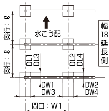
図1-11 幅18延長6本柱 幅55+18、幅60+18サイズ
