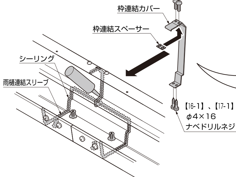
図5-10 前後枠（水下）
