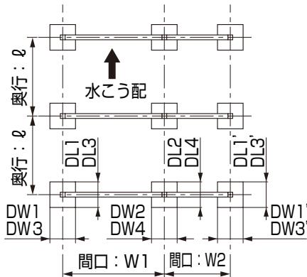
図1-5 横連棟9本柱 幅30+55、幅30+60サイズ
