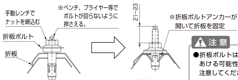
図4-9 折板ボルト取付詳細
