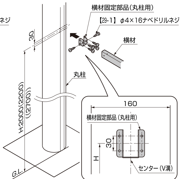
図3-4 丸柱の場合
