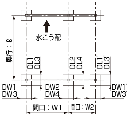
図1-4 横連棟6本柱 幅30+55、幅30+60サイズ
