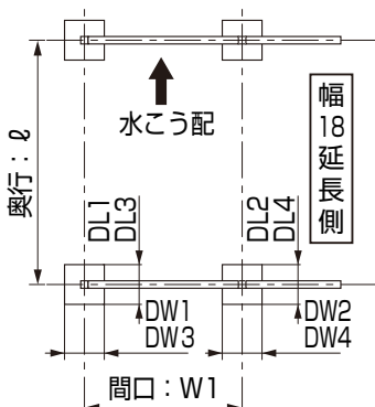
図1-10 幅18延長4本柱 幅55+18、幅60+18サイズ
