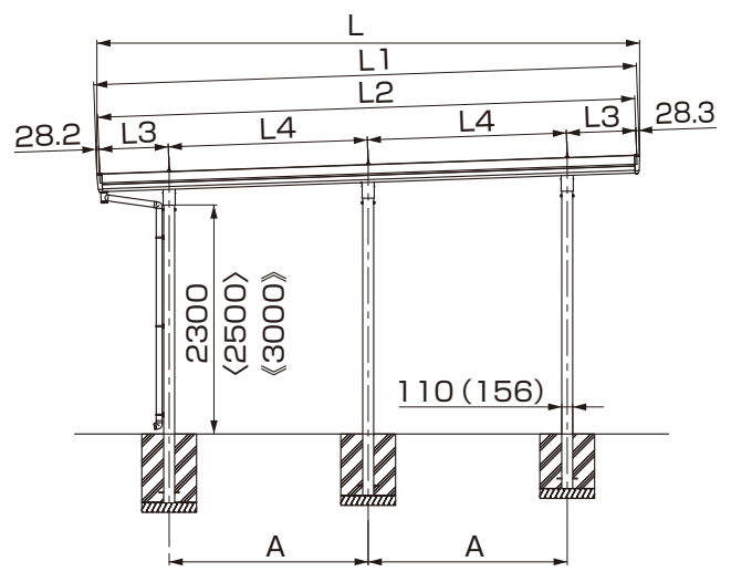
(2) 6本柱仕様
