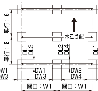
図1-8 横連棟9本柱 幅55+55、幅60+60サイズ
