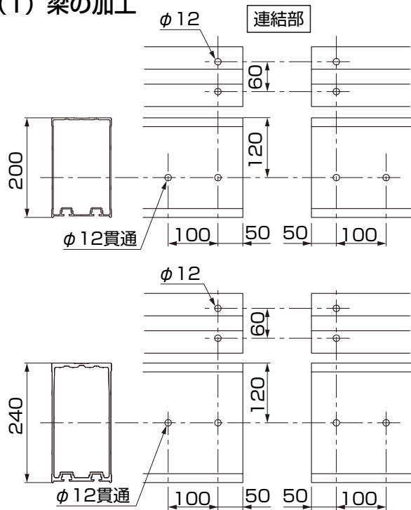
図2-9 横連棟仕様
