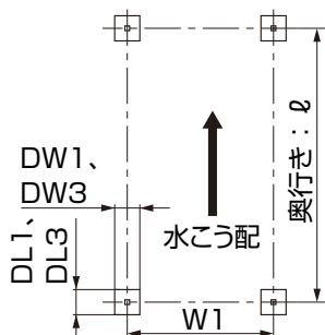
図1-1 4本柱
