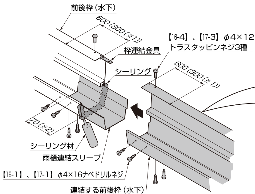
図5-6 前後枠 (水下)
