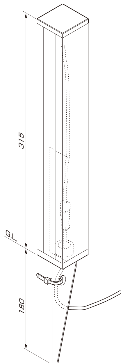
図3-2 角型
