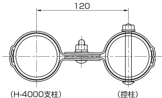
図3-1 支柱+控柱納まり図
