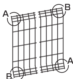
図6-1 フェンス角度:2.5°~10°
