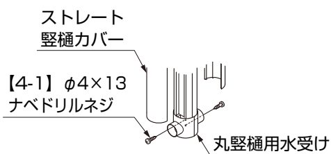
図1-8 丸柱下部
