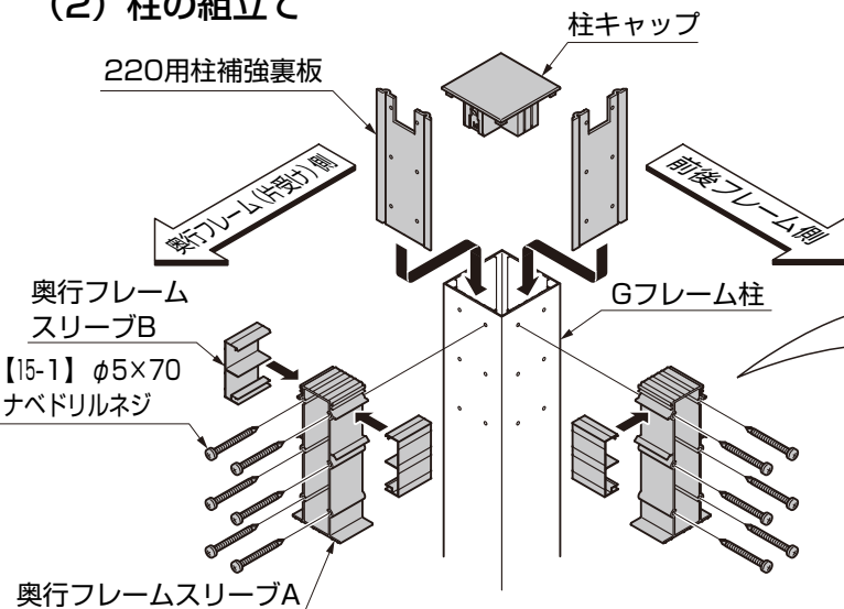
図1-11 奥行フレーム (垂木片受け) 取付部 図1-12 奥行フレーム (垂木片掛け) 取付部
