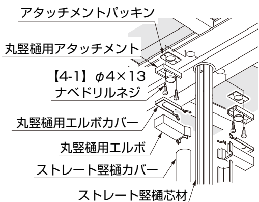
図1-7 丸柱上部
