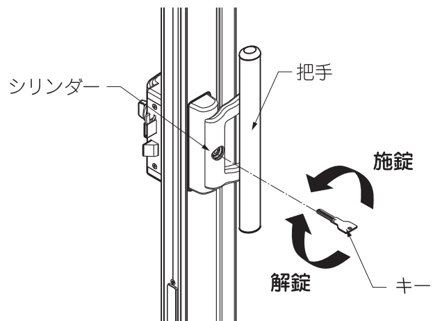
図3-2 シリンダーが右側にある場合
