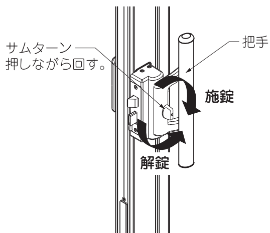
図3-3 サムターンが右側にある場合
