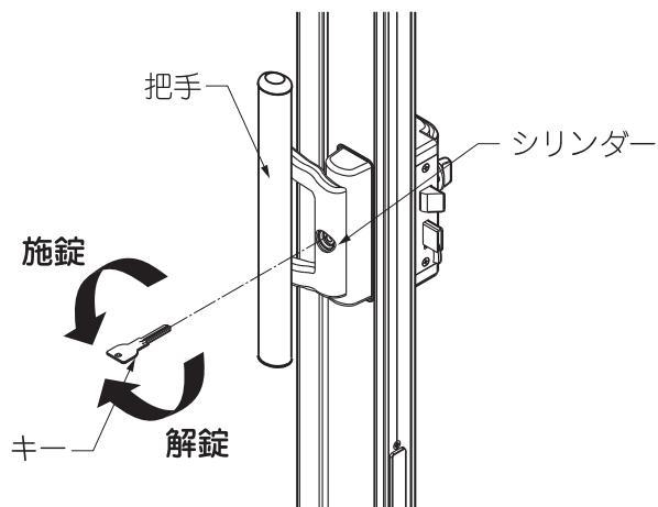
図3-1 シリンダーが左側にある場合
