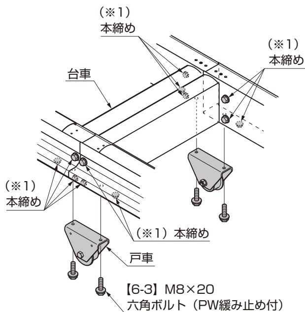
図3-2 戸車の取付け
