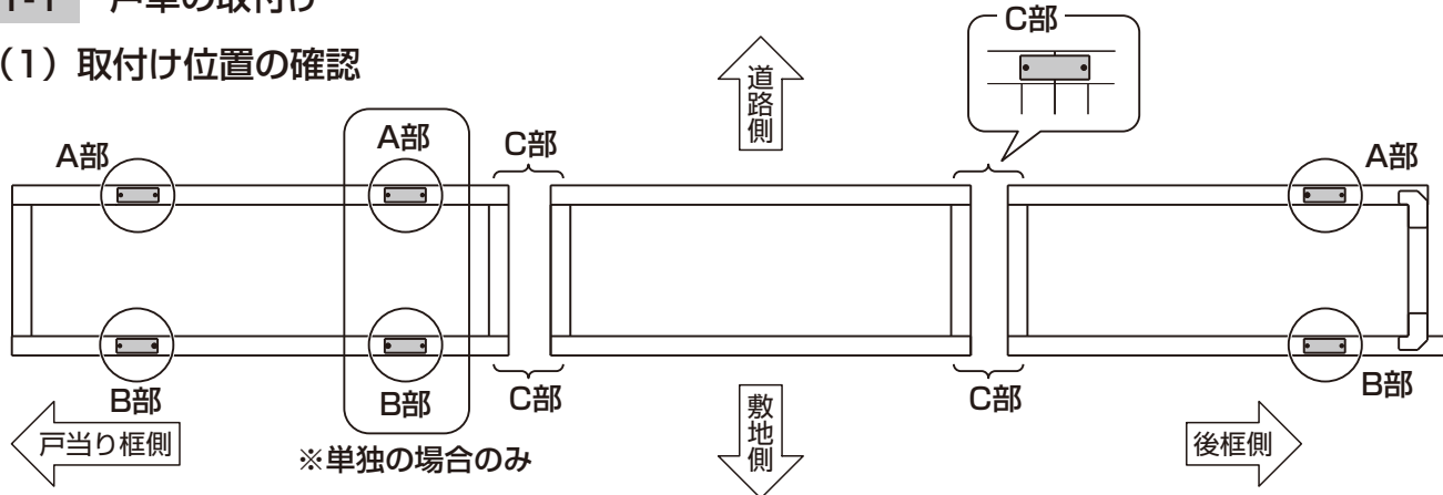
図1-1 先頭台車 戸車取付け位置 単独台車 戸車取付け位置
