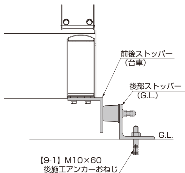
図1-2 全開時
