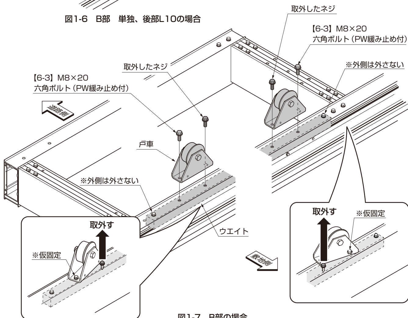
図1-7 B部の場合
