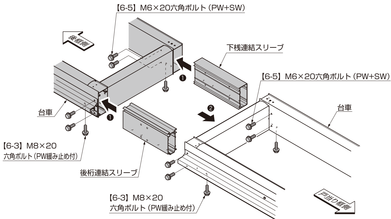
図3-1 台車の連結
