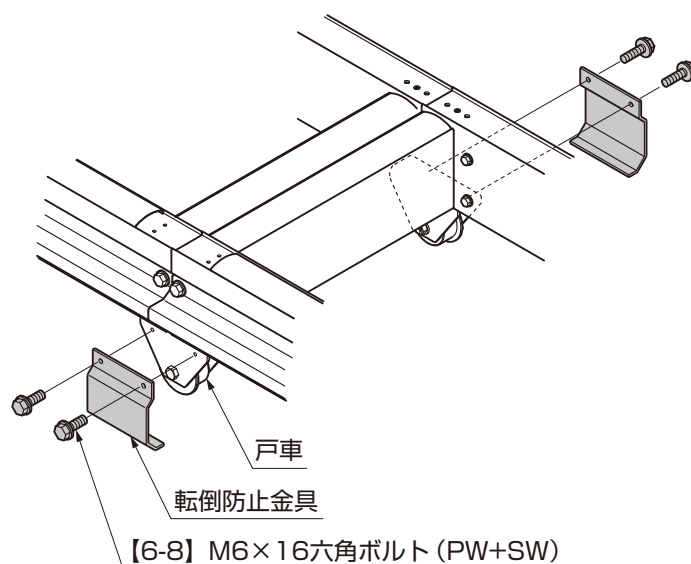
図3-3 転倒防止金具の取付け
