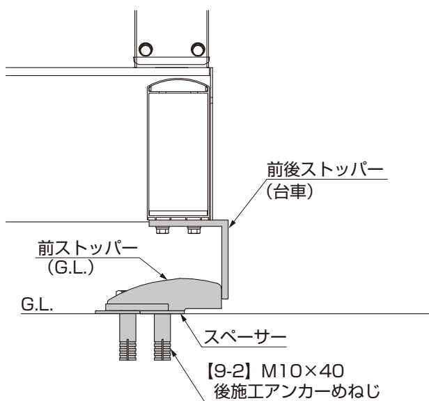
図1-1 全閉時
