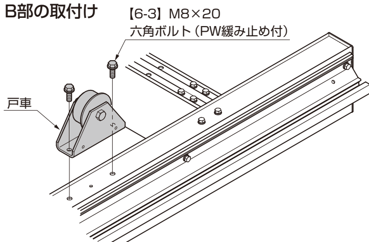
図1-6 B部 単独、後部L10の場合
