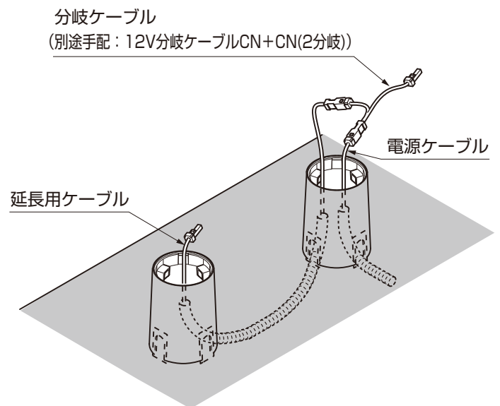
図3-2 複数灯設置の場合（コンクリートの打設）
