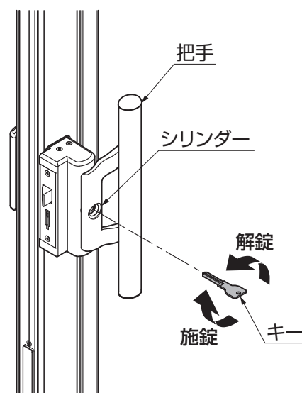
図3-4 シリンダーが右側にある場合
