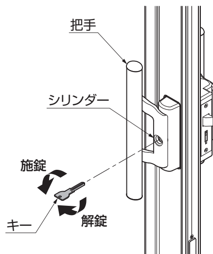
図3-2 シリンダーが左側にある場合
