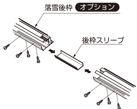
図2-7 落雪後枠1500用(オプション)の場合
