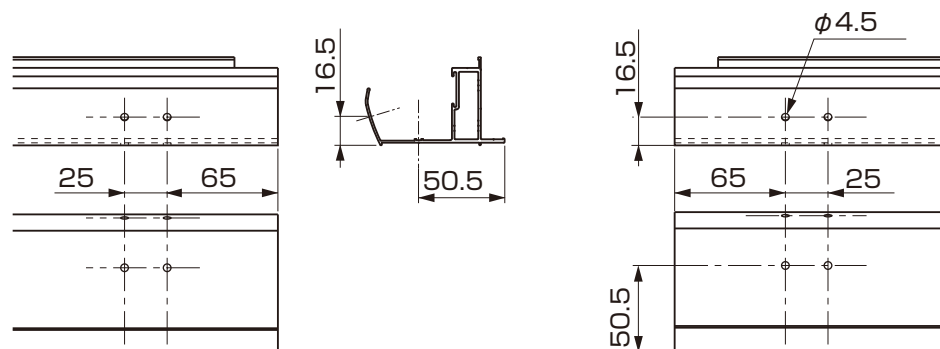
図2-4 落雪後枠 1500用 オプション の加工
