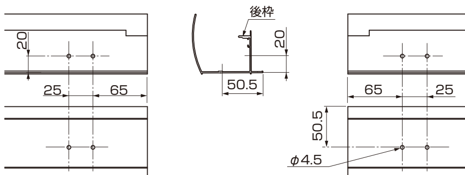
図2-1 後枠の加工
