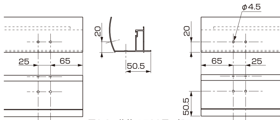
図2-3 後枠 1500用の加工
