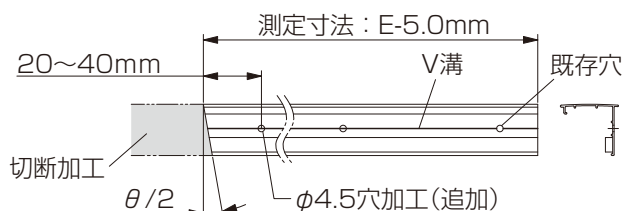
後枠側
