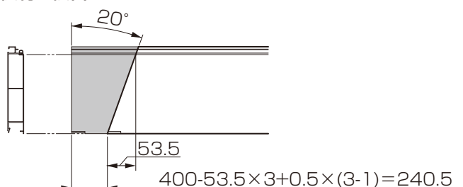
屋根材3枚目
