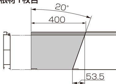
屋根材2枚目
