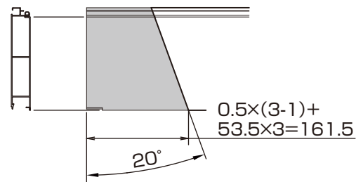
屋根材3枚目
