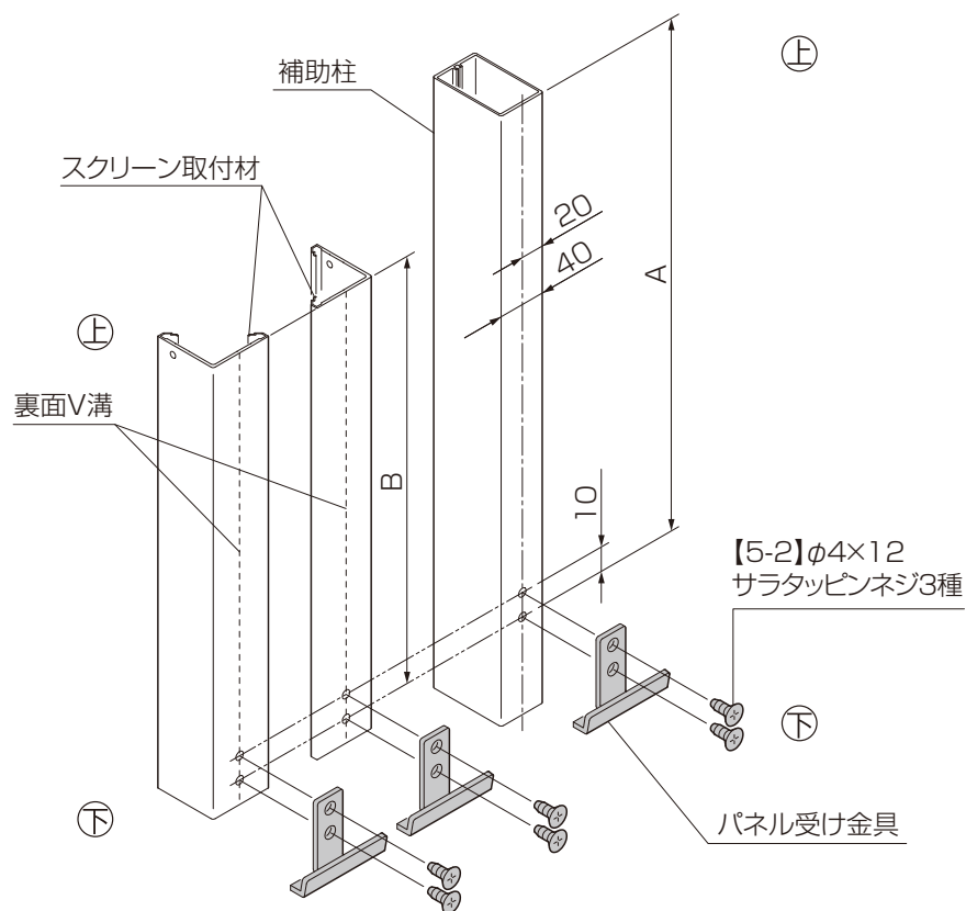
前枠側の補助柱 L1寸法
