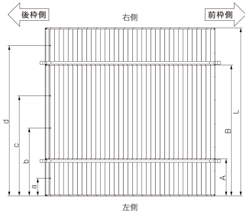
後柵固定金具の取付け位置
