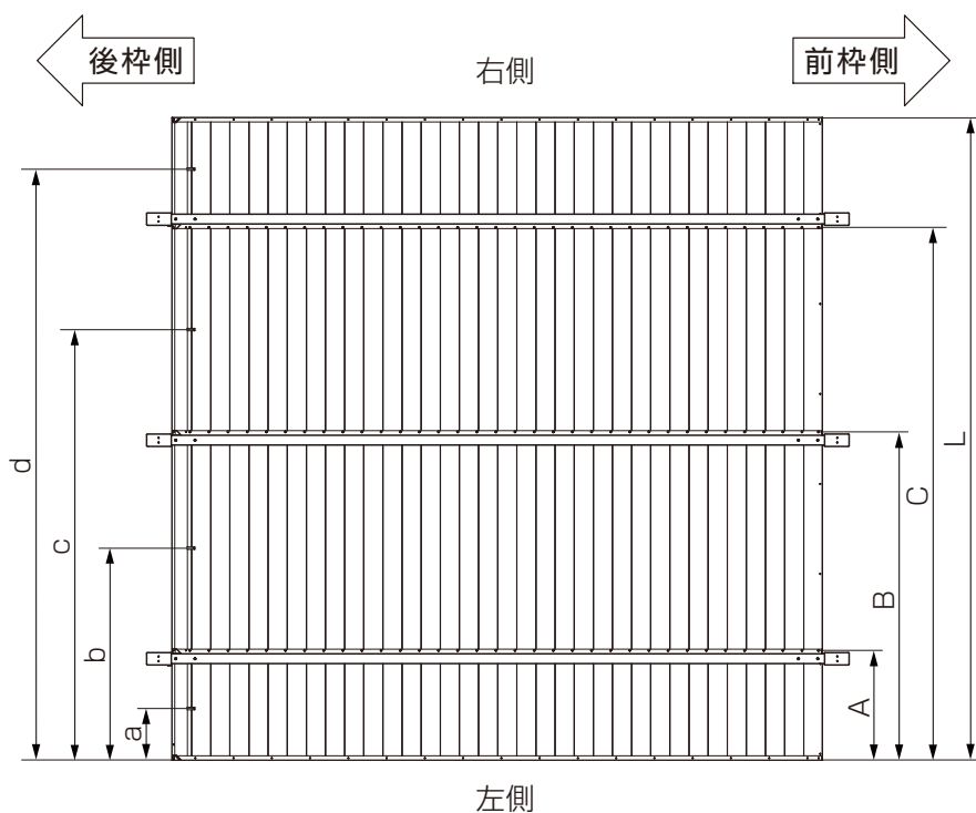
後柵固定金具の取付け位置
