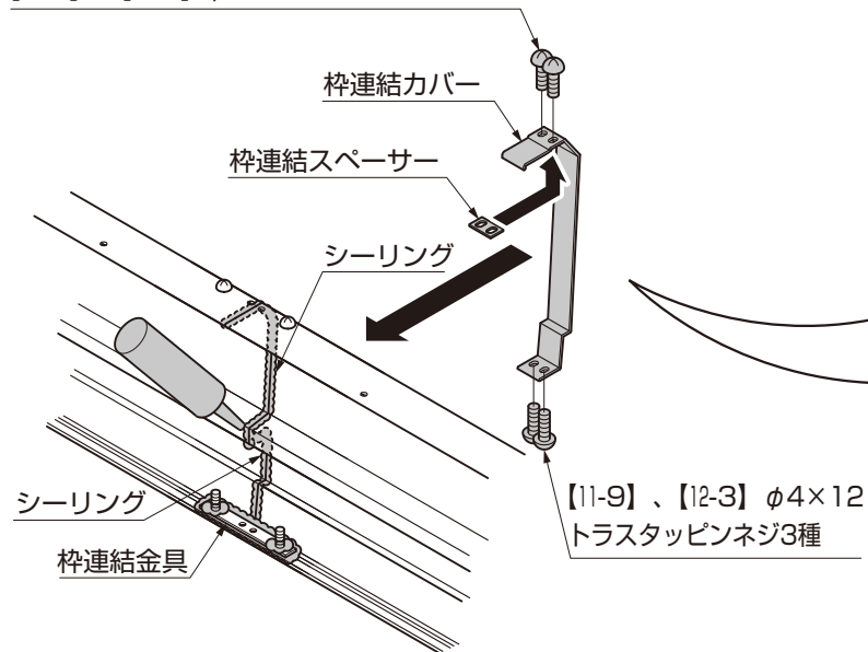
図5-8 前後枠 (水上)
