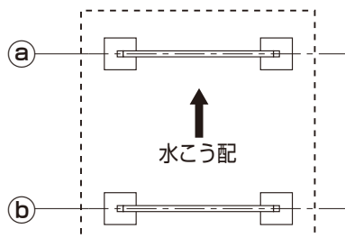
図1-16 梁2列
