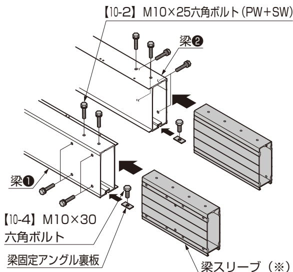
図2-16 横連棟仕様
