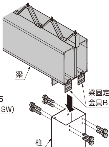
図2-13 幅80サイズの場合
