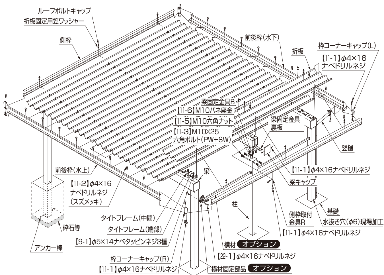
図1-1 基本仕様
