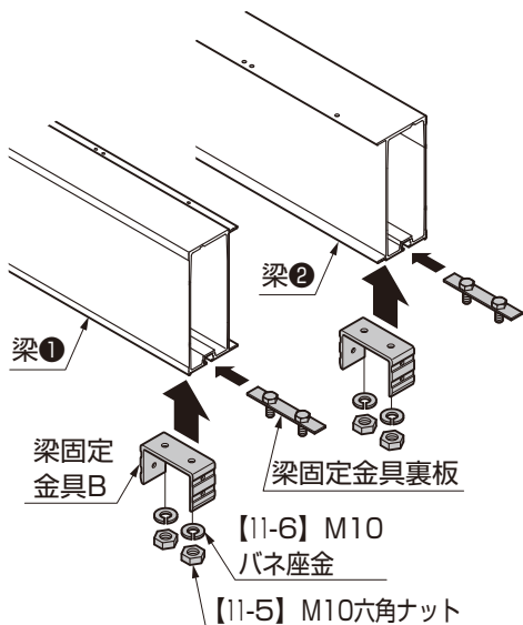
図2-9 幅55・60サイズの場合
