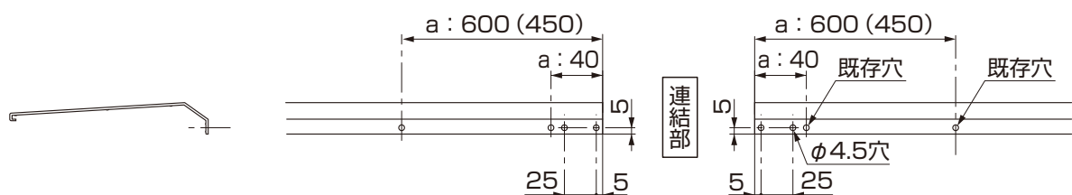
図5-3 化粧枠の加工
