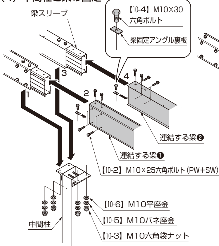
図2-20 横連棟仕様
