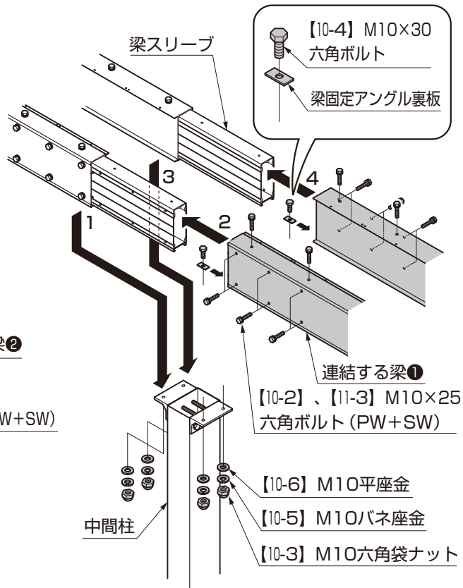
図2-21 幅18延長仕様
