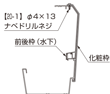
図4-4 前後枠（水下）
