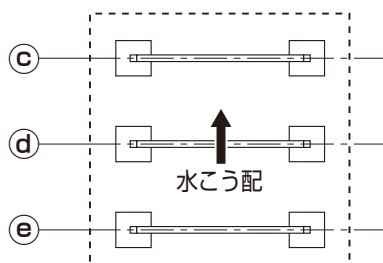
図1-17 梁3列
