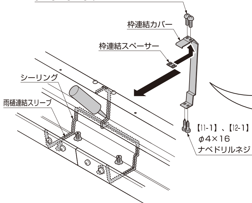
図5-10 前後枠 (水下)
