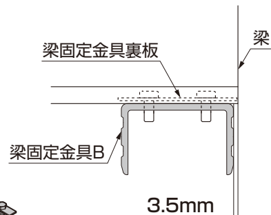
図2-11 梁固定金具B 取付け位置
