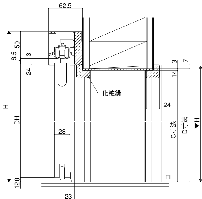
(上部化粧縁納まり)
