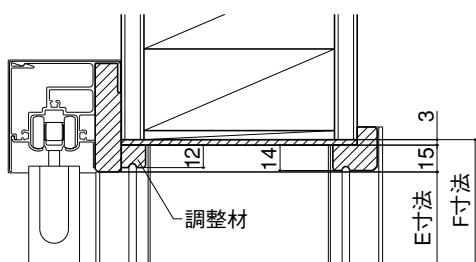
(上部化粧縁納まり)
