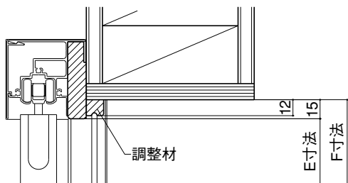
(上部化粧縁納まり)
