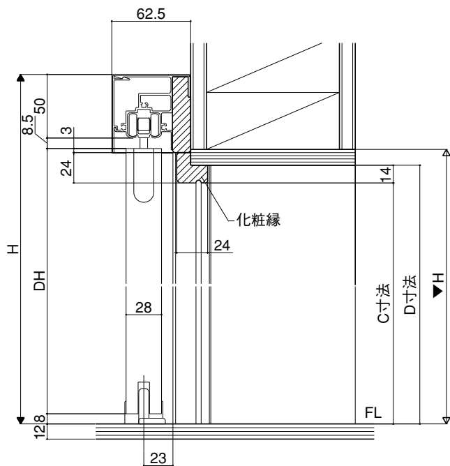
(上部化粧縁納まり)
