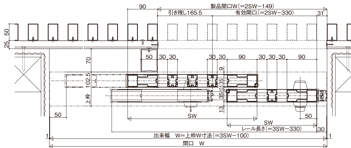
内付け袖あり片引き2枚
