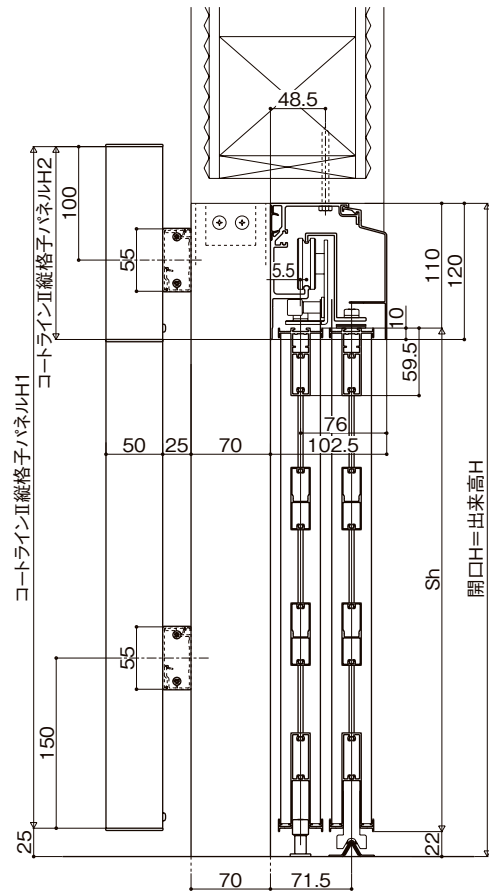
内付け袖あり片引き2枚、内付け袖あり両引き4枚
