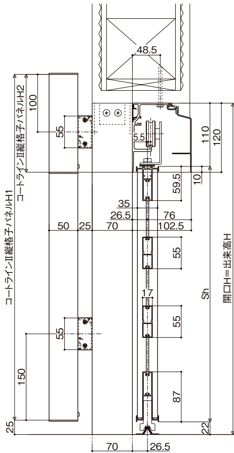
内付け袖あり片引き1枚、内付け袖あり両引き2枚
