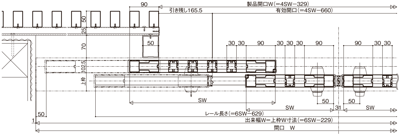
内付け袖あり両引き4枚
