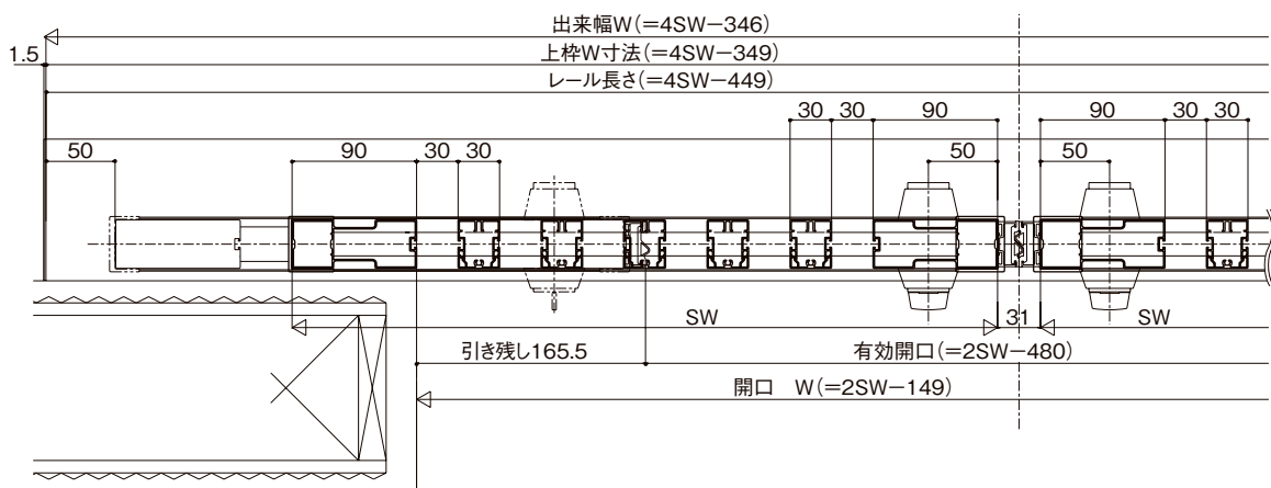
外付け袖あり両引き2枚
