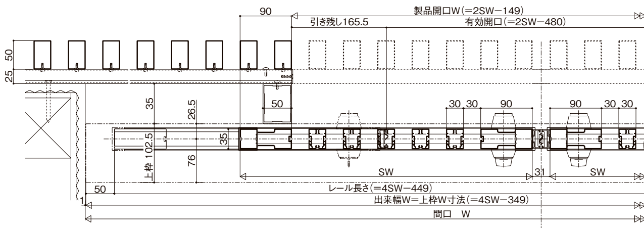
内付け袖あり両引き2枚
