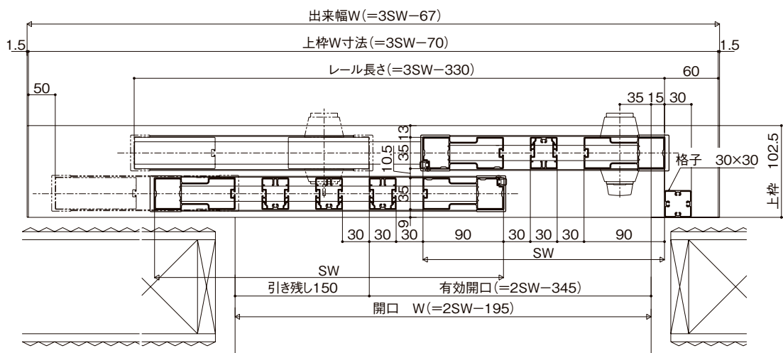
外付け袖あり片引き2枚
