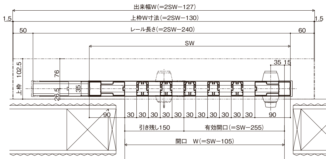
外付け袖あり片引き1枚
