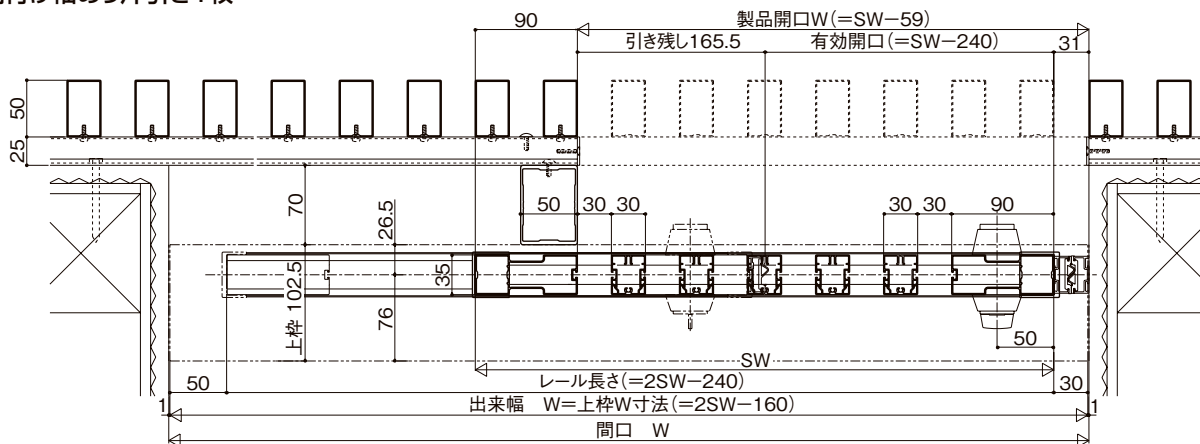
内付け袖あり片引き1枚
