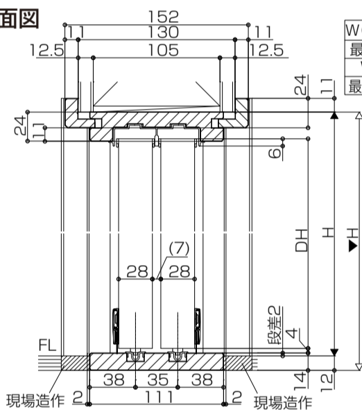
【ツバなし薄敷居納まり】
