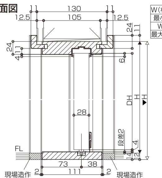
【ツバなし厚敷居納まり】
