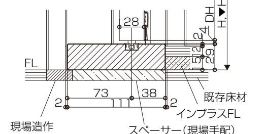
【ツバなし厚敷居納まり】
