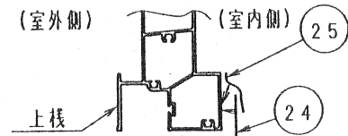
②④ 取説貼付詳細図
