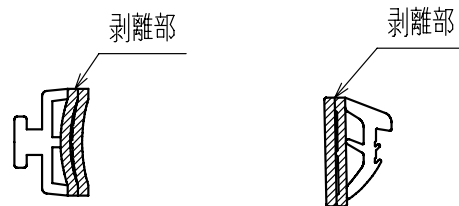
先付けビード
