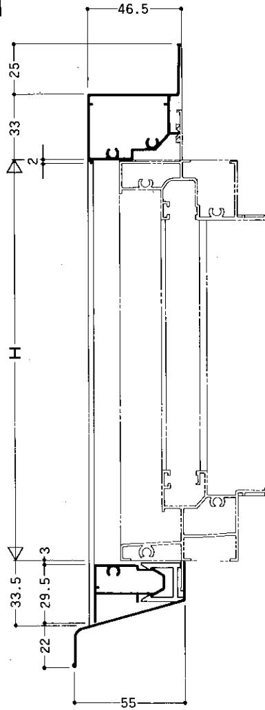
● 縦断面図
