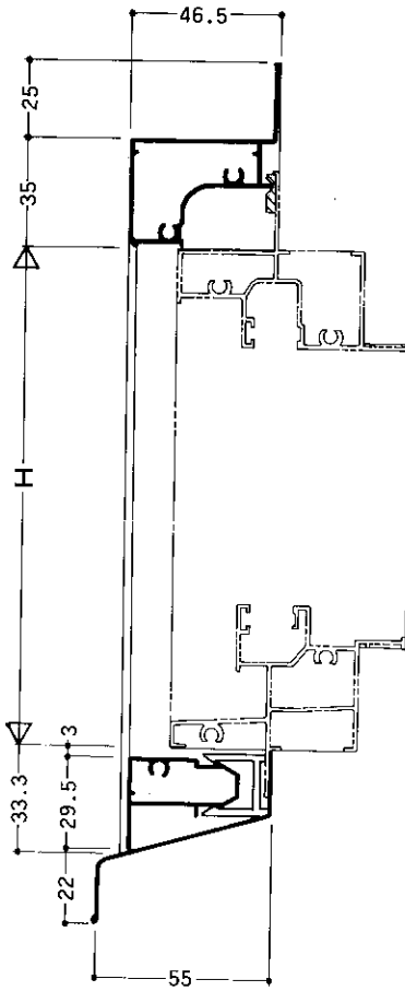
● 縦断面図
