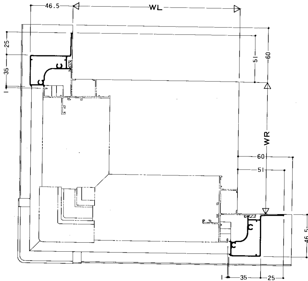
● 横断面図
