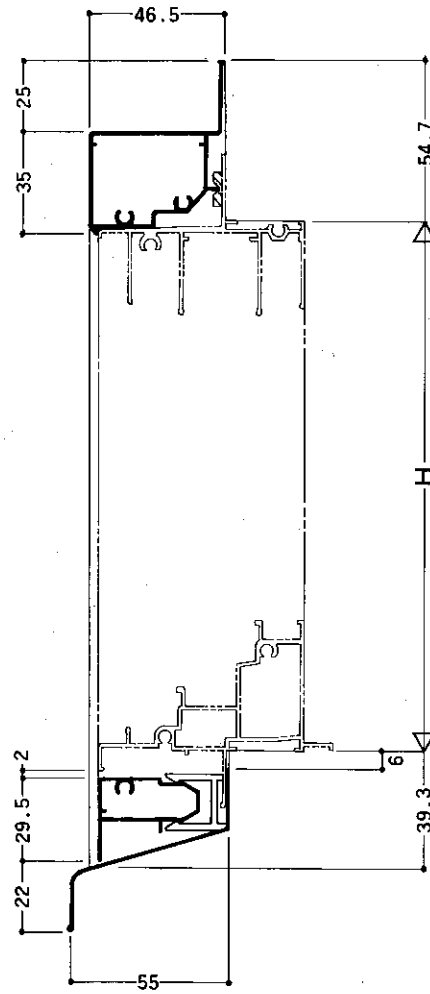
● 縦断面図
