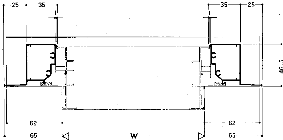
● 横断面図
