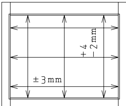
内法寸法
